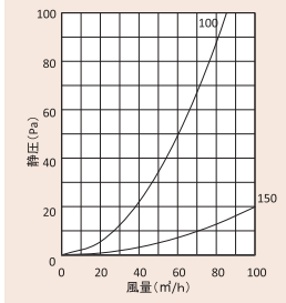
圧力損失特性
